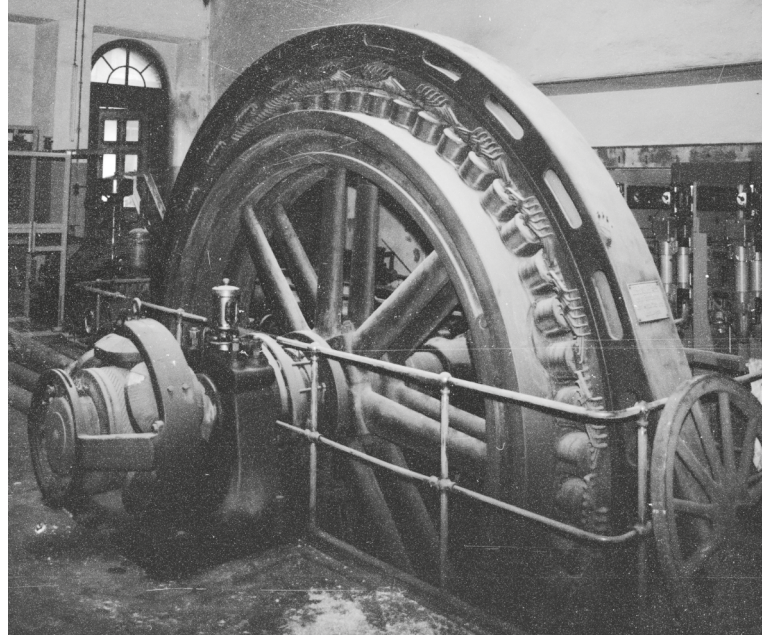
Gaswerk Schlieren, Sulzer Dampfmaschine 1904, Hans-Peter Bärtschi 1998, e-pics.ethz.ch
